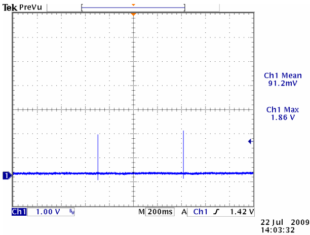
Vin=48V
