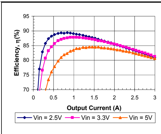
V_o = 1.2V
