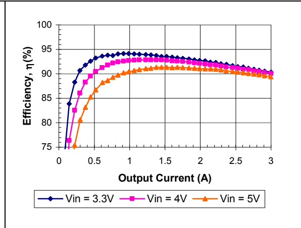
V_o = 2.5V
