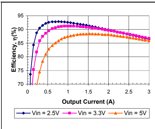
V_o = 1.8V
