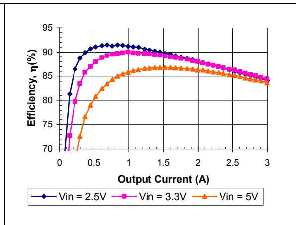
V_o = 1.5V
